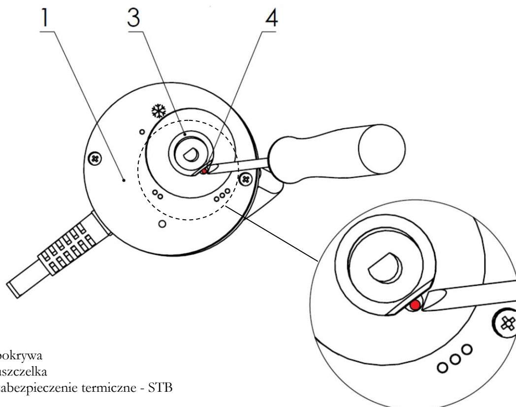
Rys.4 Demontaż pokrętła grzałki – umieszczenie wkrętaka w szczelinie.
