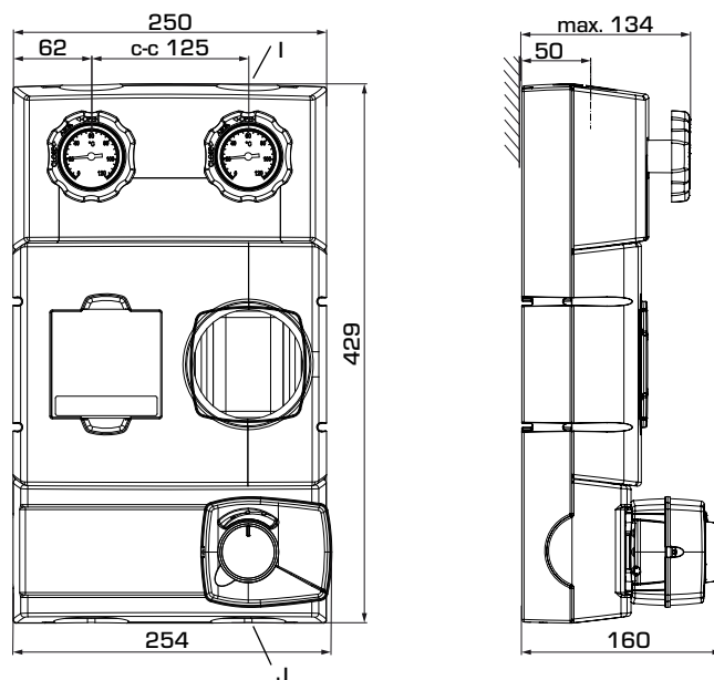
GRF221
