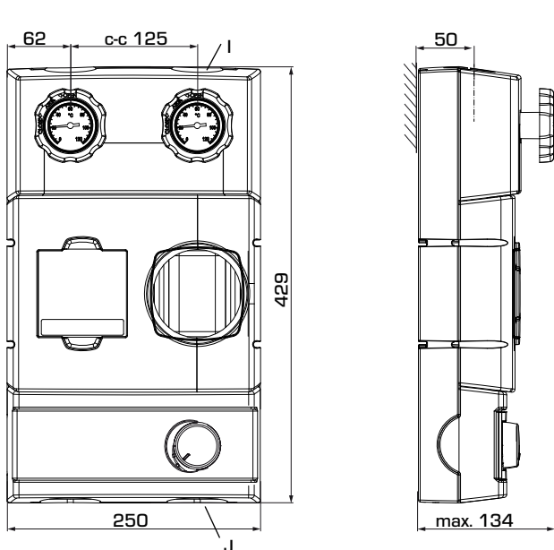
GRF211
