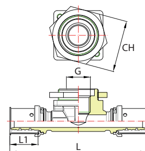
TEE FEMALE FOR CONNECTION TO LAVATORY FLUSH-WATER TANK / RACCORDO A T FLANGIATO FEMMINA PER CASSETTA DI RISCIAQUO
